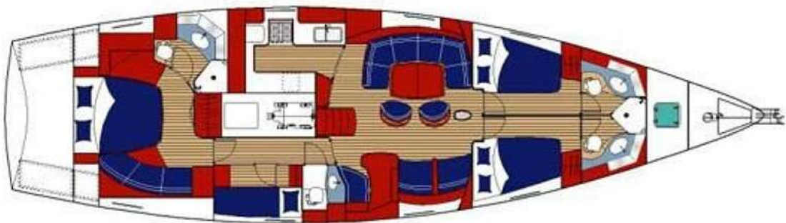
Version 1 cabine propriétaire arrière - 1 cabine coursive - 2 cabines avant 1 owner aft cabin - 1 watch cabin - 2 forward cabins version
